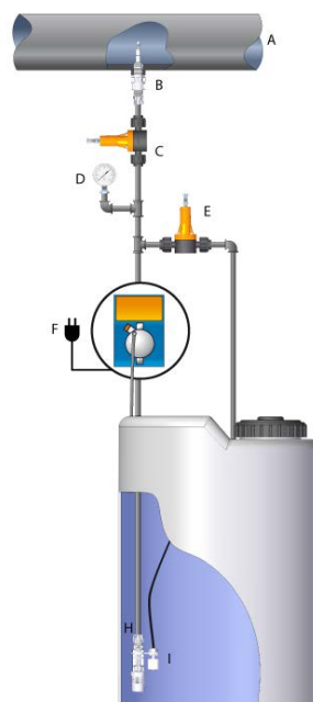
Fig. 6 - Planta típica
