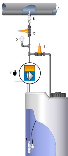
Fig.5 – Azionamento spurgo per adescamento
