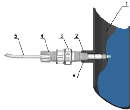
Fig. 7 - Montaggio Raccordo
